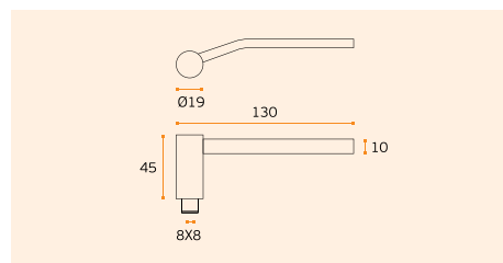
IN.00.054 Material: EN 1.4301 - Satinado / Satin / Satin RB08M - Roseta standard / Standard rose
