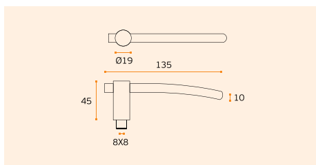
IN.00.053 ONE Material: EN 1.4301 - Satinado / Satin / Satin RB08M - Roseta standard / Standard rose
