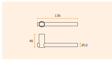
MV.00.001 TUBYK Material: EN 1.4301 - Satinado / Satin / Satin RB08M - Roseta standard / Standard rose Design: Miguel Vasconcelos
