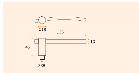
IN.00.051 Material: EN 1.4301 - Satinado / Satin / Satin RB08M - Roseta standard / Standard rose
