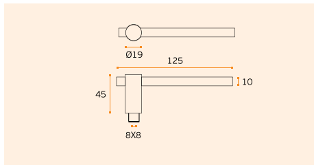
IN.00.050 Material: EN 1.4301 - Satinado / Satin / Satin RB08M - Roseta standard / Standard rose
