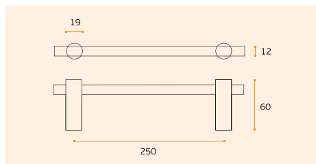
MV.07.030 TUBYK Material: EN 1.4301 - Satinado / Satin / Satin Asa de porta / Door handle / Manillone de puerta Design: Miguel Vasconcelos
